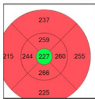
OD ILM-RPE Thickness
